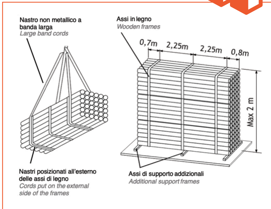
STOCCAGGIO / HANDING STORAGE
